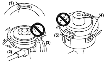
Рис. 20 Осмотр триммерной головки
